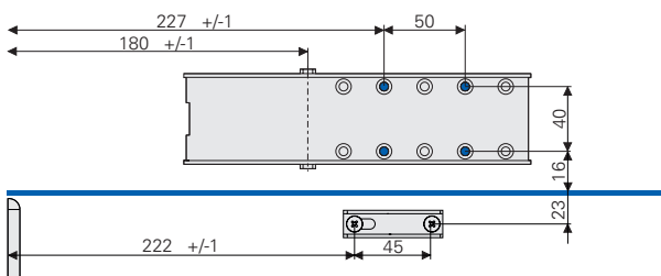
Closing force EN 3
