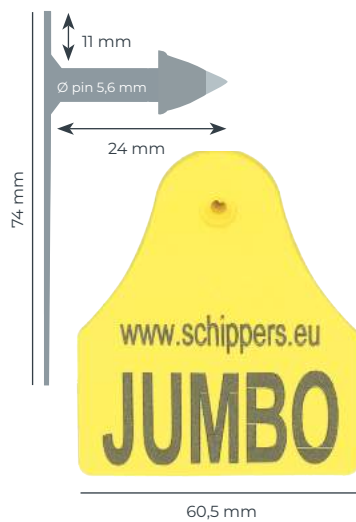
MS Tag Jumbo (Robust pin)
