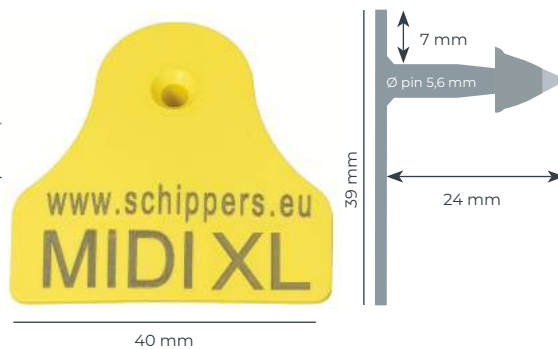
MS Tag Midi XL (Robust pin)
