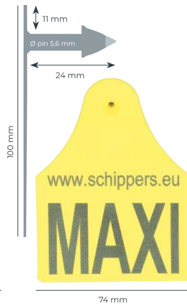
MS Tag Maxi (Robust pin)
