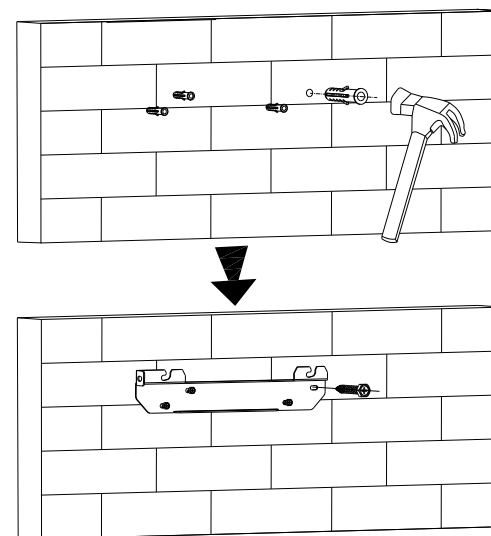
Slika 5.8 Šematski dijagram instalacije zidnog nosača
