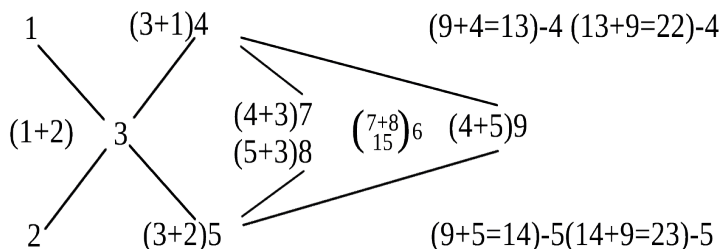
Fig. 2. Generarea aritmetică a primelor nouă numere
