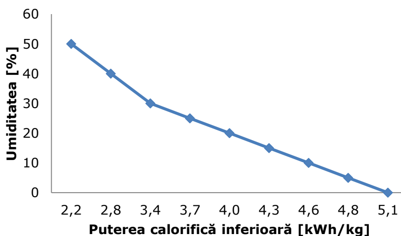
Puterea calorică în raport cu umiditatea
