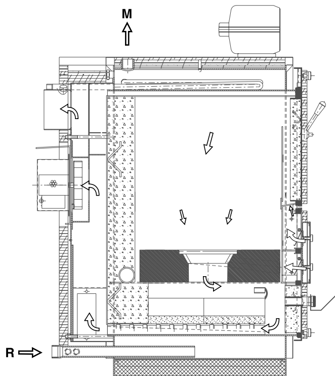
M = Tur apăcaldă R = Retur instalație P = Aer primar S = Aer secundar F = Gaze de ardere
