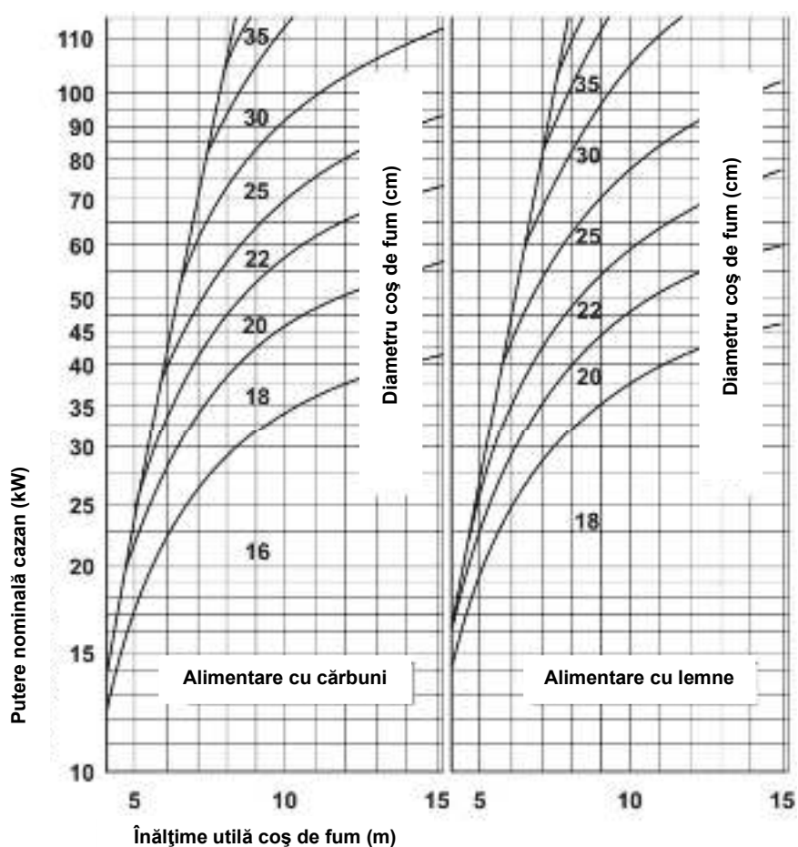
Figura 5. Dimensiunile coșului de fum pentru cazanele DOMINUS
