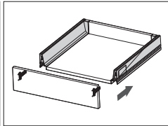
Turn screw driver to release the drawer front / Rotiți șurubelnița pentru a elibera partea frontală a sertarului
