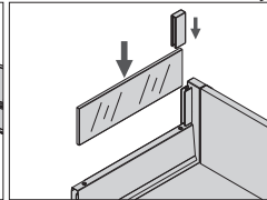
Side assembly / Montaj laterală
