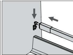
Fit the front / Fixați partea frontală
