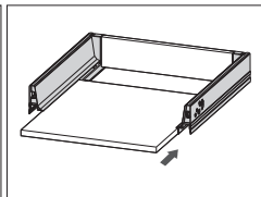
Bottom assembly / Montaj bază
