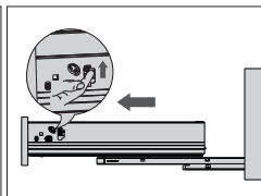
Lift the release handle and Pull out the drawer / Ridicați mânerul de deblocare și trageți sertarul
