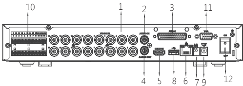
DH-XVR7116HE-4KL-X
