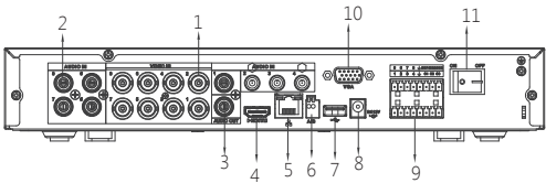
DH-XVR7108HE-4KL-X
