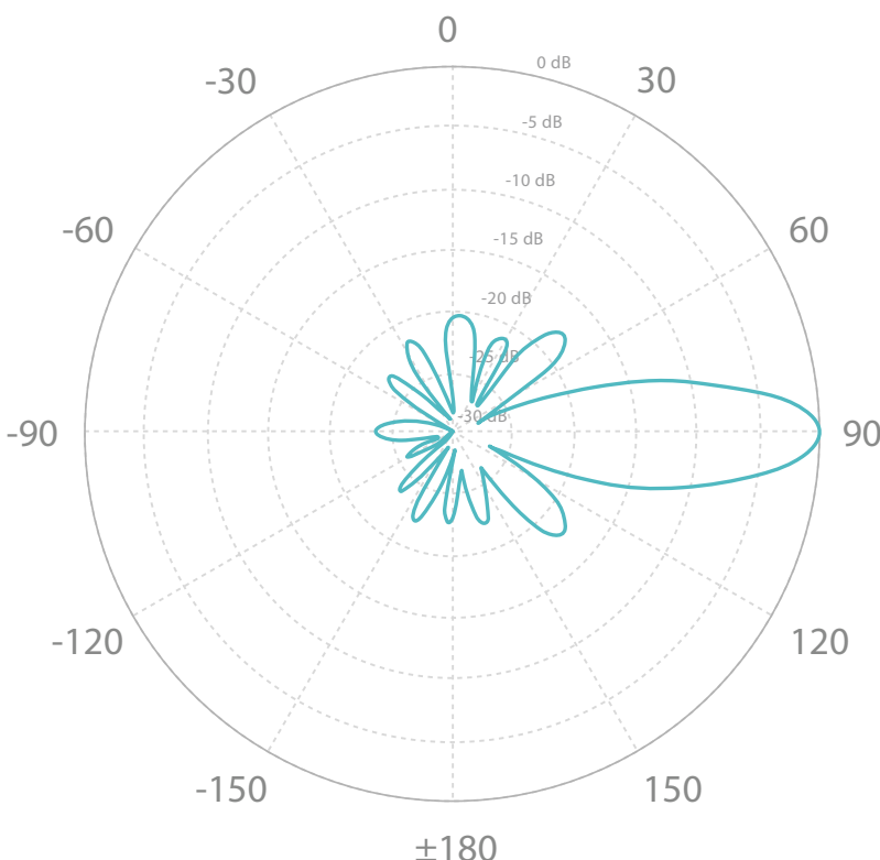
Elevation
