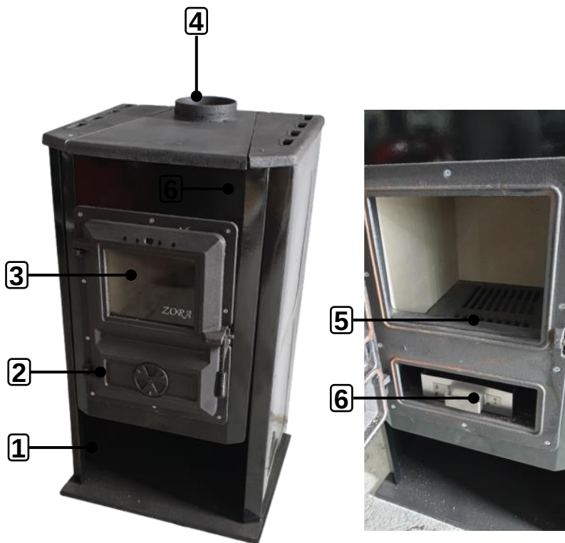
Lista componentelor
