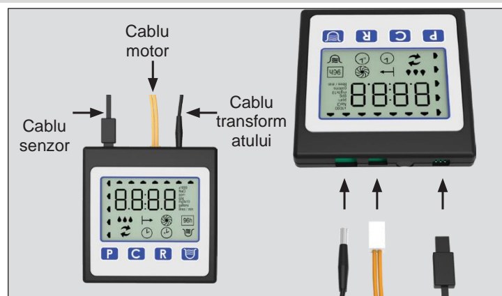
Figura 9: Conectarea panoului de comanda
