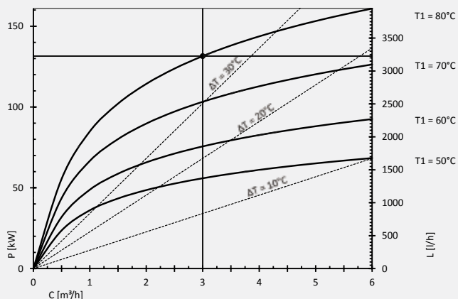
Diagrame de performanță Storatherm Aqua Heat Pump 500/1 pt. temperatura de 45°C
