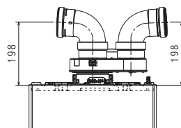
CONDUCTE DIVIZATE Ø80-80 mm CU ADAPTOR
