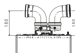
CONDUCTE DIVIZATE Ø80-80 mm CU ADAPTOR COMPACT
