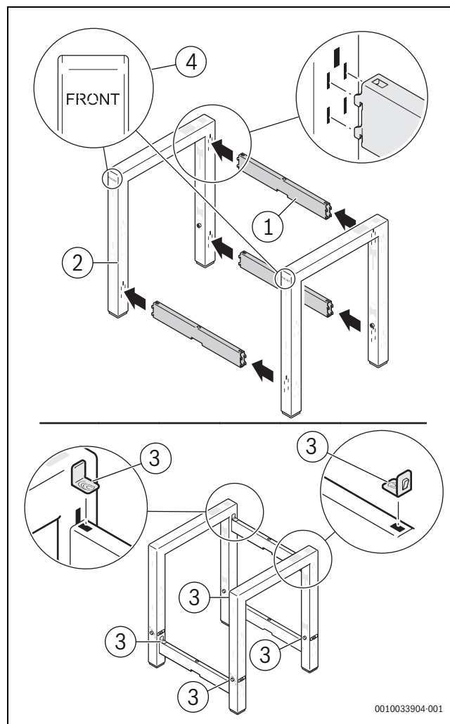
Fig. 8 Instalarea cadrului
