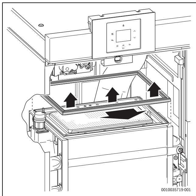
Fig. 41 Îndepărtarea garniturii arzătorului
