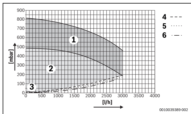
Fig. 51 Înălțimea de refulare a pompei GB272-50
