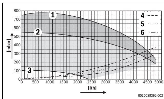
Fig. 54 Înălțimea de refulare a pompei GB272-100
