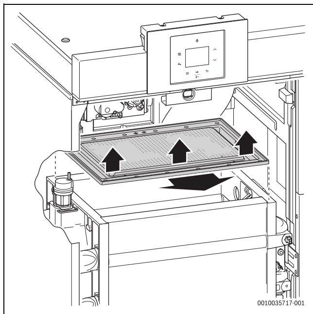
Fig. 42 Îndepărtarea arzătorului
