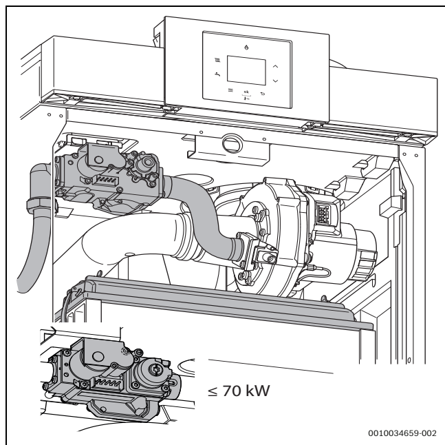
Fig. 35 Inspectarea traseului gazului
