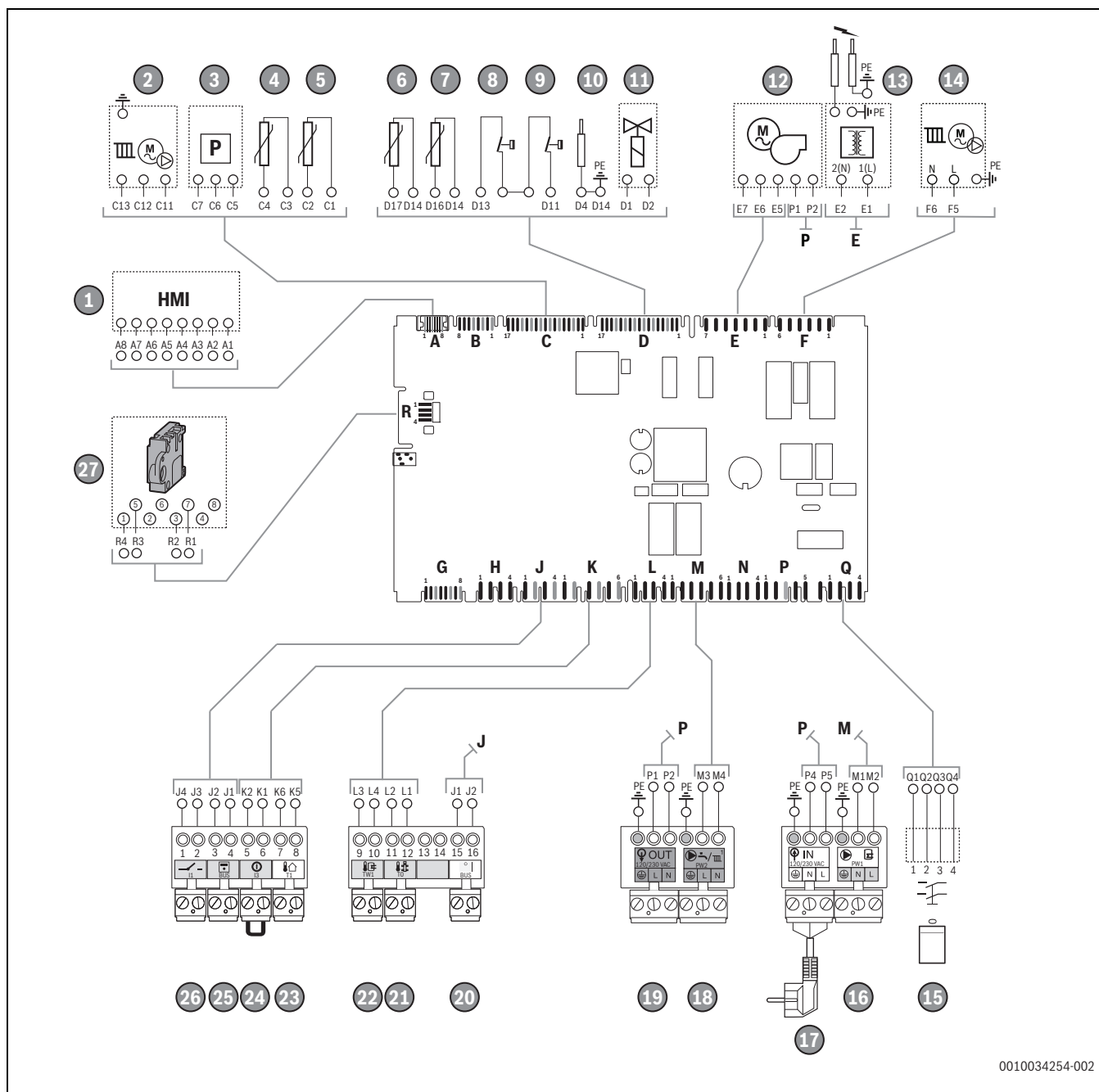
Fig. 50 Schemă electrică
