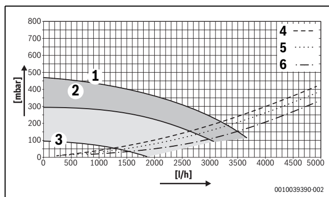
Fig. 52 Înălțimea de refulare a pompei GB272-70
