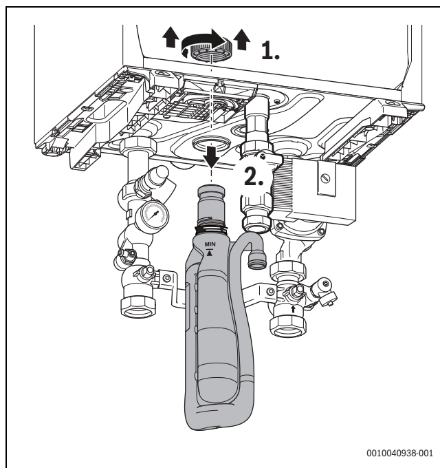
Fig. 44 Scoateți sifonul cazanului
