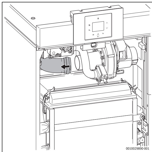
Fig. 38 Îndepărtarea conductei de admisie a aerului
