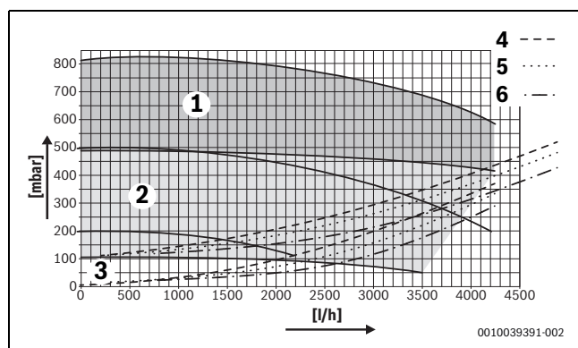
Fig. 53 Înălțimea de refulare a pompei GB272-85
