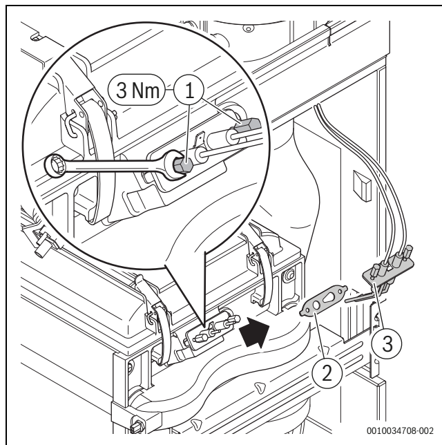
Fig. 47 Introducerea aprinzătorului de gaz
