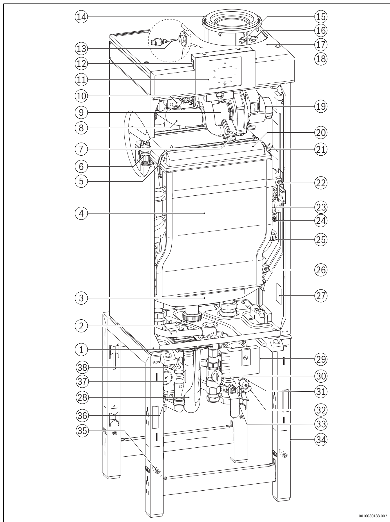
Fig. 1 GB272 cu set de racordare pe cadru
