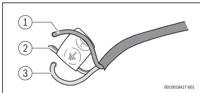
Fig. 31 Montarea ștecherului
