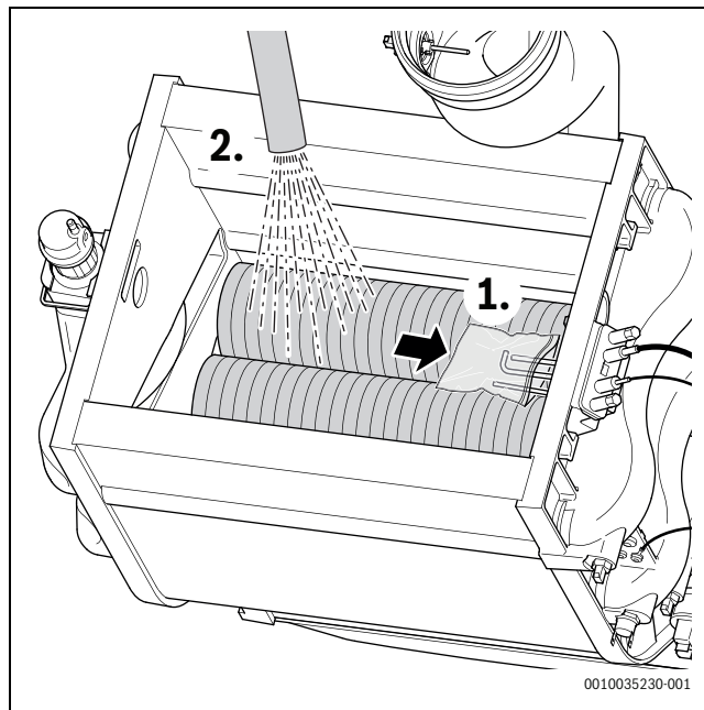
Fig. 43 Curățarea schimbătorului de căldură
