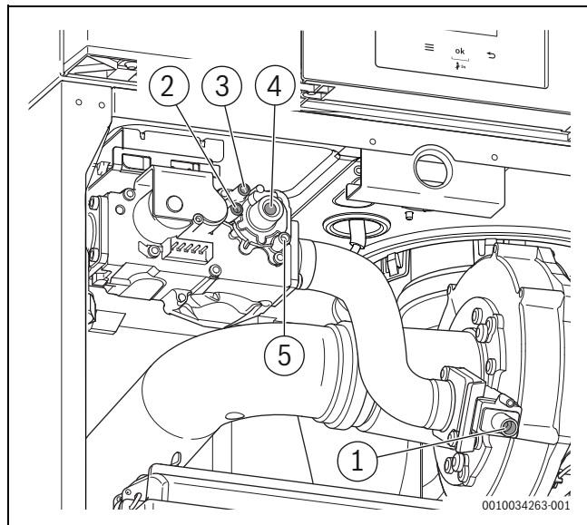
Fig. 33 Prezentare generală a orificiilor de testare și a șuruburilor de reglare ≥ 85 kW
