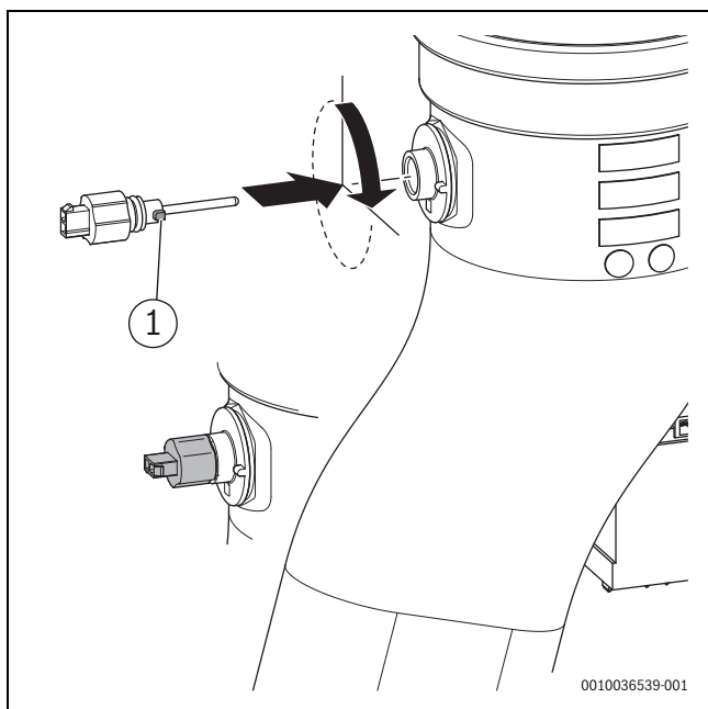
Fig. 48 Înlocuirea senzorului de temperatură a gazelor arse
