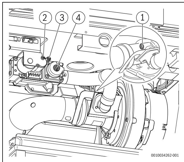
Fig. 32 Prezentare generală a orificiilor de testare și a șuruburilor de reglare ≤ 70 kW
