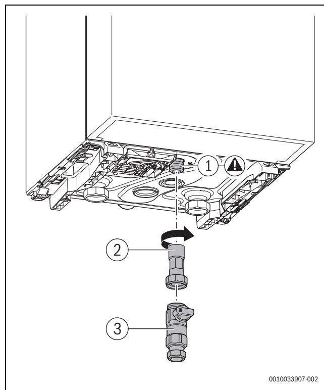
Fig. 13 Instalarea vanei de gaz
