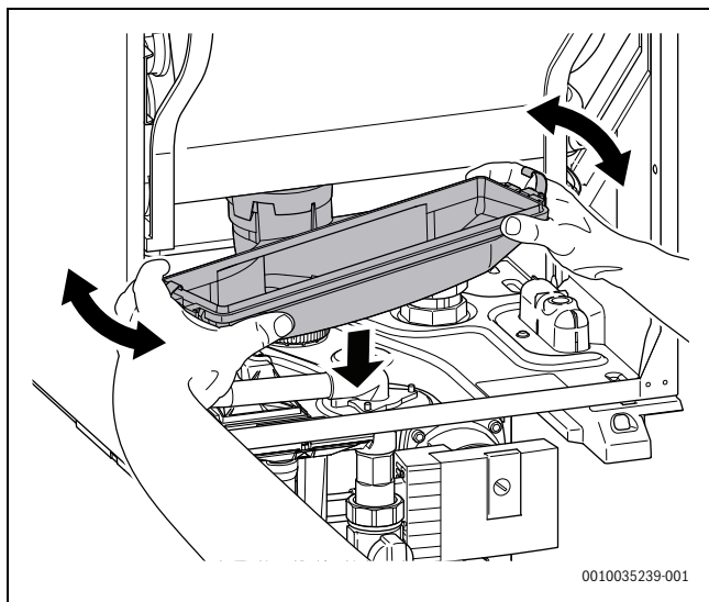
Fig. 46 Scoateți recipientul pentru condensat.
