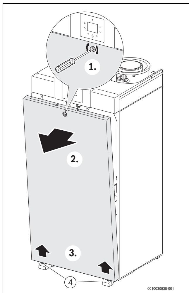
Fig. 6 Deschiderea peretelui frontal
