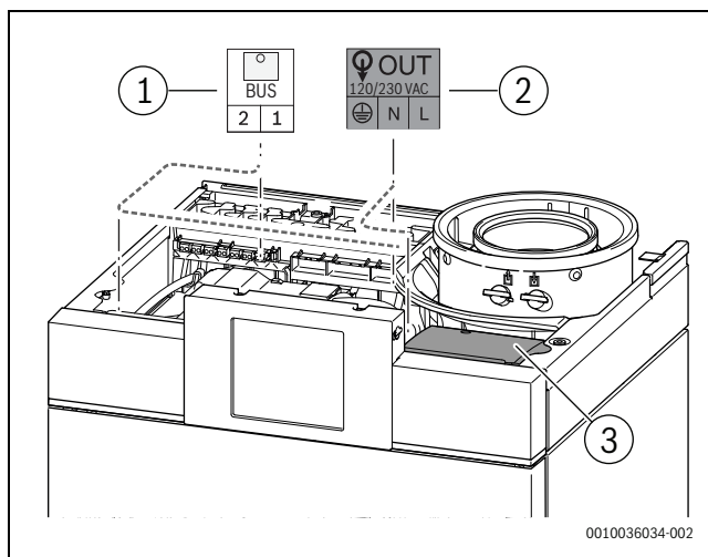
Fig. 30 Montarea modului funcțional
