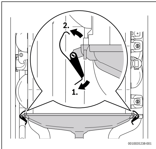
Fig. 45 Deschideți elementele de fixare ale recipientului pentru condensat
