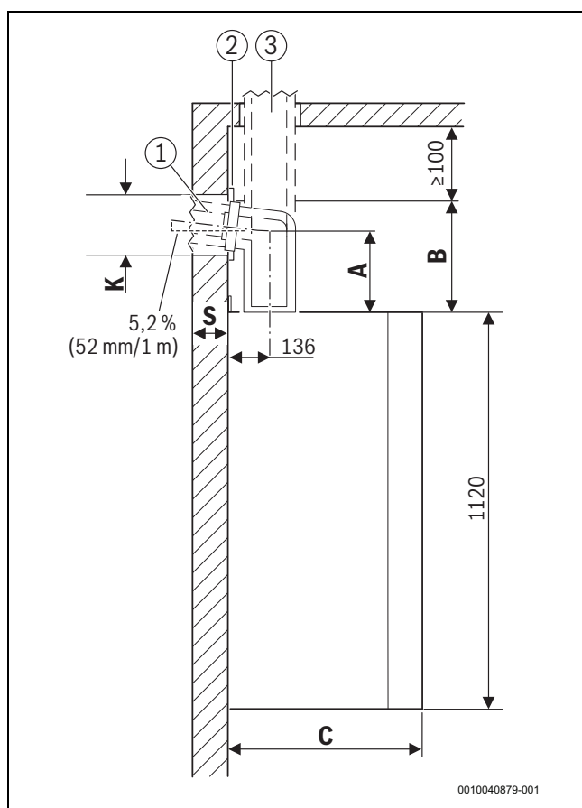
Fig. 4 Vedere laterală [mm]
