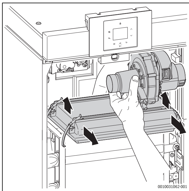
Fig. 40 Îndepărtați unitatea de gaz-aer împreună cu capacul arzătorului.
