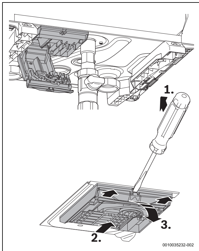
Fig. 25 Deschiderea unității terminale a pompei
