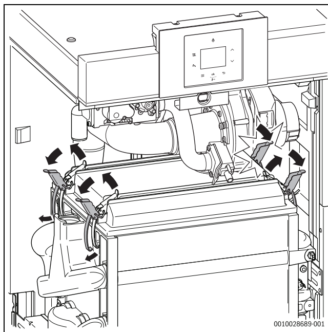
Fig. 39 Deschideți elementele de fixare
