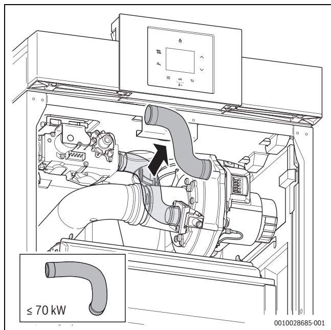
Fig. 37 Îndepărtați furtunul de gaz \geq 85 kW
