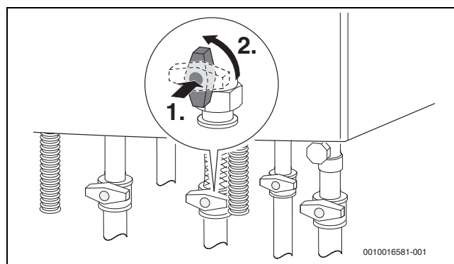
Fig. 3 Deschiderea robinetului de gaz
