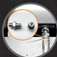
Valvă siguranță anti-explozie pentru sistemul hidraulic
