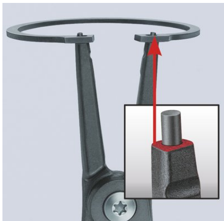
Cleștele de precizie KNIPEX pentru inele de siguranță: montajul fără torsiune, ușor și rapid al inelului
