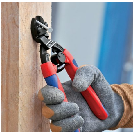
cap angular la 20° cu eclisă pe o parte și tăiere laterală pentru tăiere coplanară, cu spațiu liber pentru apucare
