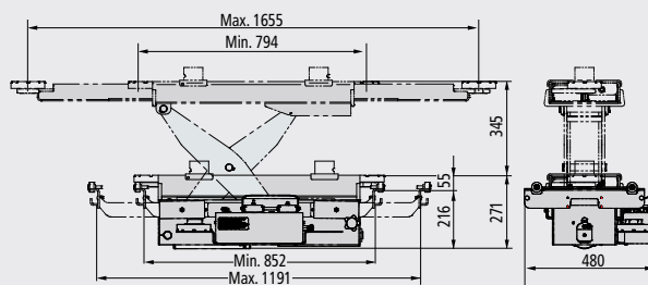
J40PXL
