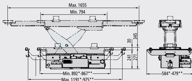
J40PRL* - JS40PRL**
