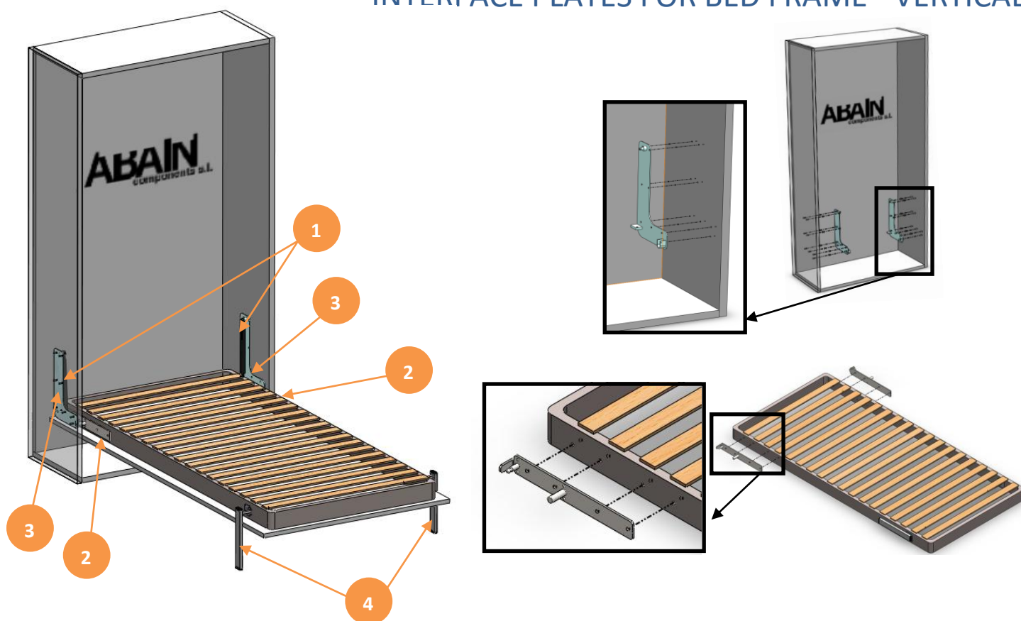
1. Elevadores a gas con retención en bajada / Gas lifts with lowering retention
