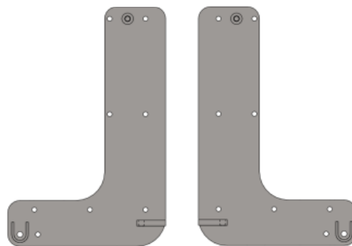
4. Sugerencia de patas de apoyo al suelo / Suggested legs support to the ground
