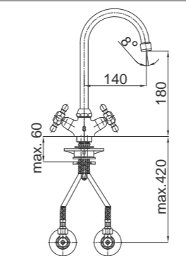
STIL - ARMATURA ZA UMIVALNIK ARMATURA ZA UMIVAONIK BASIN MIXER
