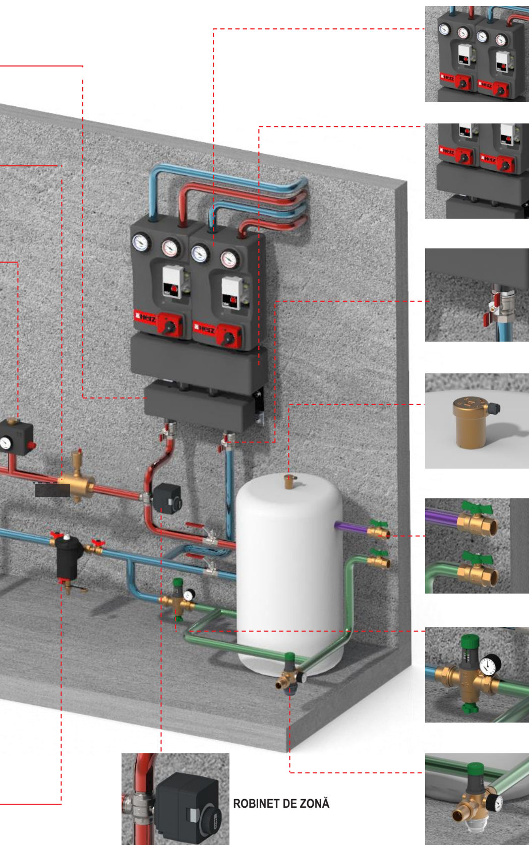
Grup de pompare MIX
