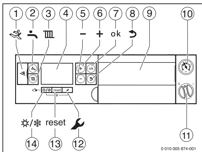
Fig. 36 Panou de comandă la capacul deschis al panoului de comandă
