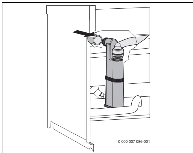
Fig. 28 Montarea furtunului la sifonul pentru condensat
