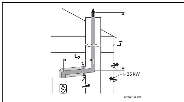
Fig. 20 Ghidarea rigidă a gazelor arse în puț conform B 33 cu alimentare cu aer dependentă de aerul din încălț prin ghidarea concentrică a aerului/gazelor arse în încăperea centralei termice
