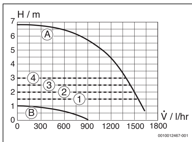
Fig. 86 Câmpuri caracteristice ale pompei și linii caracteristice ale pompei
