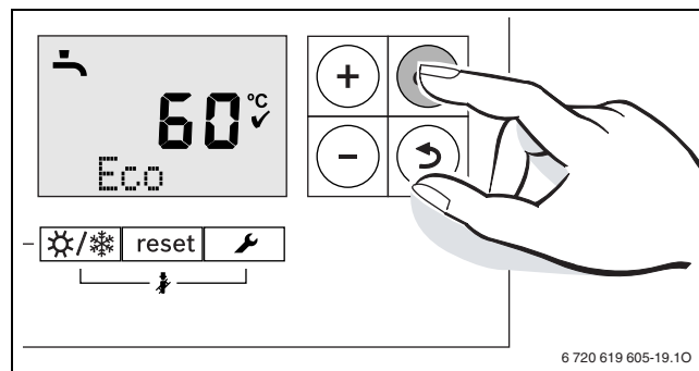
Fig. 45 Confirmare afășaj temperatură apă caldă
