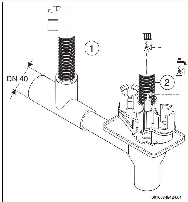
Fig. 30 Montarea furtunului pentru condensat și a furtunului supapei de siguranță la sifon
