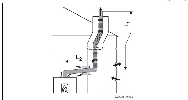
Fig. 19 Ghidarea flexibilă a gazelor arse în puț conform B 23p /B 53p cu alimentare cu aer dependentă de aerul din încălț la nivelul aparatului și elementului de legătură concentric dintre încăperea centralei termice și puț
