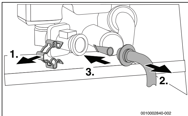
Fig. 57 Demontați sita din țeava pentru apă rece
