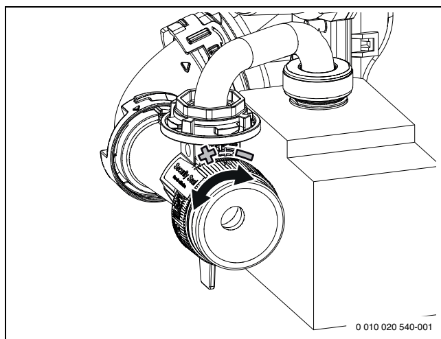
Fig. 50 Setarea raportului între gaz și aer
