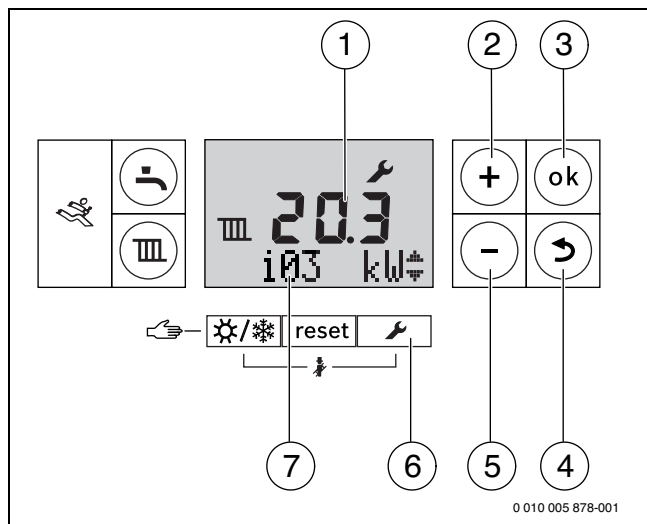
Fig. 49 Privire de ansamblu asupra elementelor de comandă
