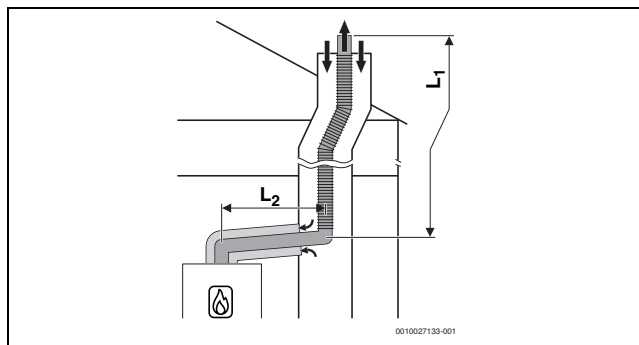
Fig. 17 Ghidarea flexibilă a gazelor arse în puț conform C_{93x} și ghidarea concentrică a aerului/gazelor arse în încăperea centralei termice
