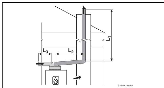
Fig. 12 Ghidarea rigidă a gazelor arse în puț conform C_{53} și ghidarea aerului/gazelor arse cu țevi separate pentru alimentarea cu aer și evacuarea gazelor arse în încăperea centralei termice
