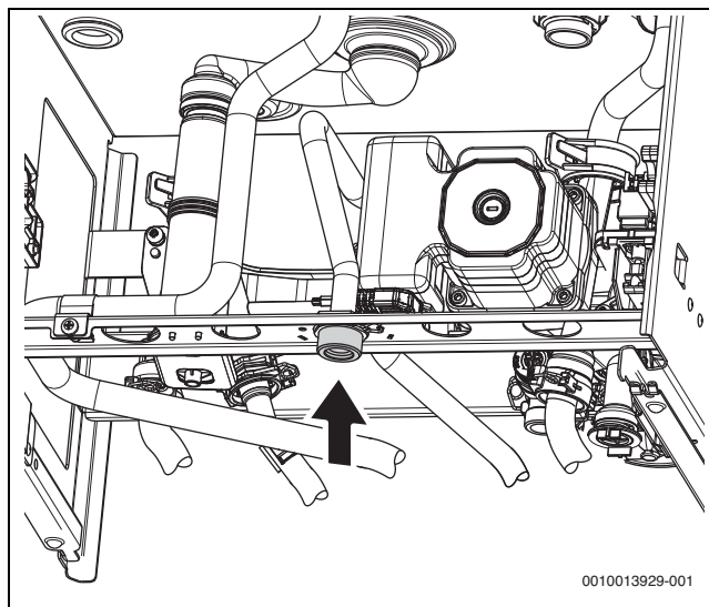
Fig. 24 Racord vas de expansiune exterior
