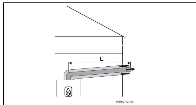
Fig. 7 Ghidarea concentrică, orizontală a aerului/gazelor arse conform C 13x prin peretele exterior
