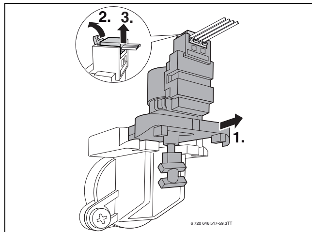
Fig. 72 Demontarea motorului vanei cu 3 căi
