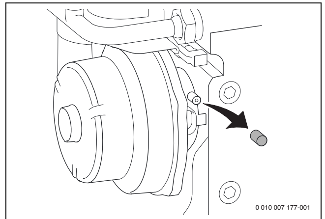
Fig. 63 Orificiu de măsurare la sistemul de amestecare
