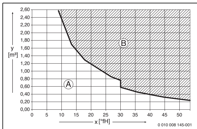
Fig. 23 Cerințe privind apa de alimentare și completare în °fH pentru aparate < 50 kW
