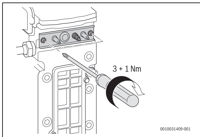
Fig. 59 Remontarea setului de electrozi
