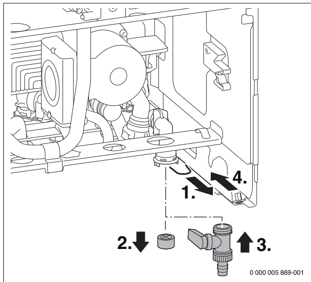
Fig. 29 Montarea robinetului de alimentare și golire
