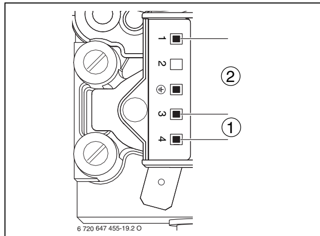
Fig. 74 Punctele de măsurare la vana de gaz
