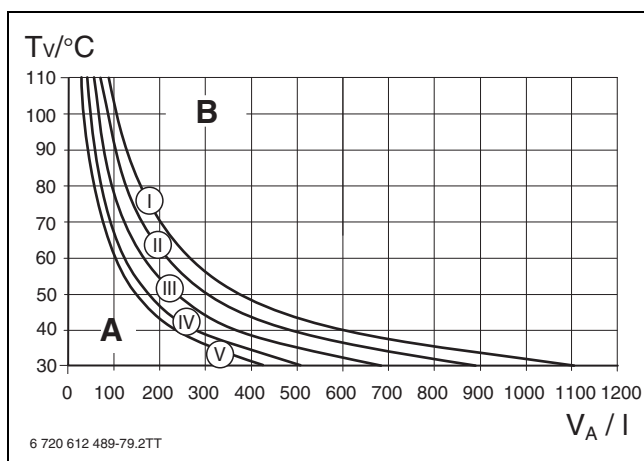
Fig. 25 Curbele caracteristice ale vasului de expansiune
