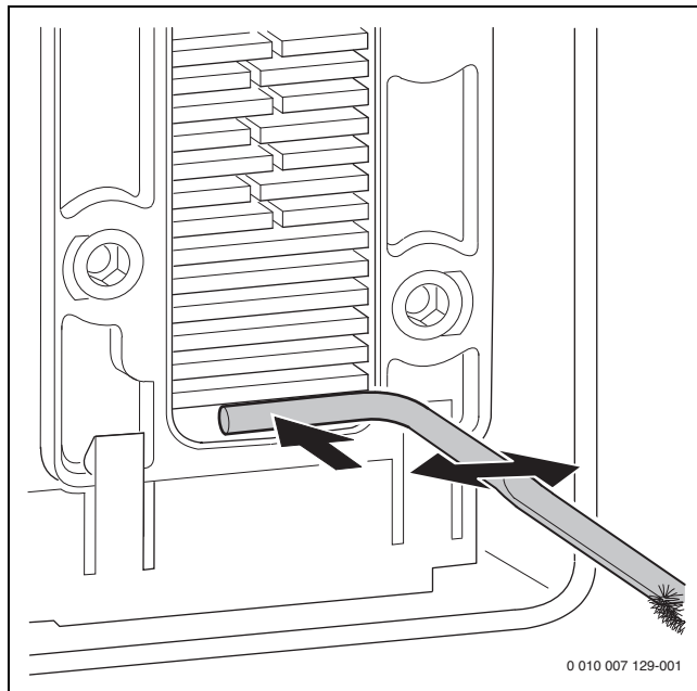
Fig. 67 Curățarea recipientului pentru condensat
