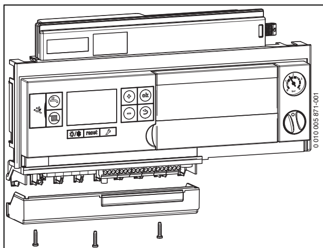
Fig. 34 Îndepărtarea capacului
