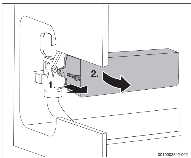
Fig. 56 Demontarea schimbătorului de căldură în plăci
