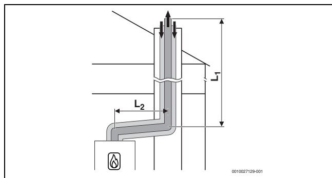
Fig. 8 Ghidarea concentrică a aerului/gazelor arse în puț conform C_{33x}
