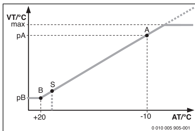
Fig. 85 Curbă de încălzire
