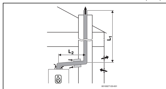
Fig. 18 Ghidarea rigidă a gazelor arse în puț conform B 23p /B 53p cu alimentare cu aer dependentă de aerul din încălțată la nivelul aparatului și elementului de legătură concentric dintre încăperea centralei termice și puț
