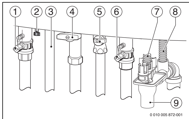
Fig. 31 Racorduri pe partea de gaz și apă (accesorii)
