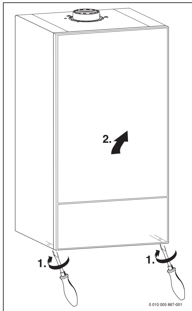
Fig. 26 Scoaterea mantalei
