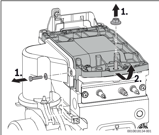
Fig. 61 Slăbirea capacului arzătorului
