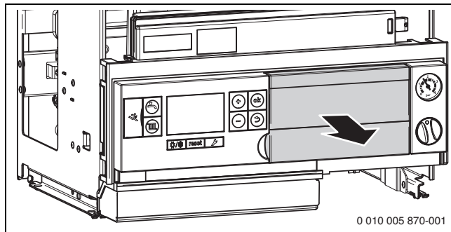
Fig. 33 Îndepărtarea acoperirii și montarea unității de comandă
