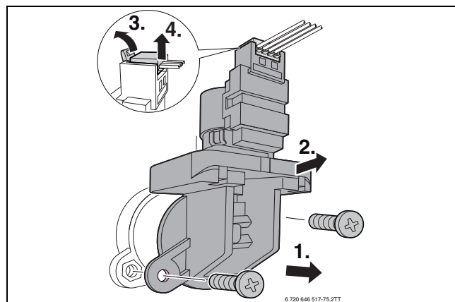
Fig. 73 Demontarea vanei cu 3 căi
