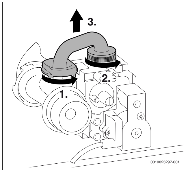
Fig. 75 Demontarea țevii de gaz
