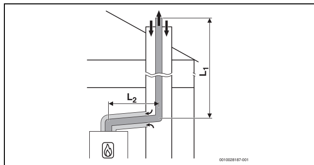
Fig. 16 Ghidarea rigidă a gazelor arse în puț conform C_{93x} și ghidarea concentrică a aerului/gazelor arse în încăperea centralei termice
