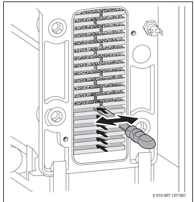
Fig. 64 Lama de curățare
