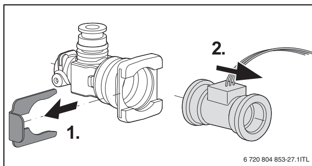
Fig. 58 Demontați turbina de pe țeava pentru apă rece
