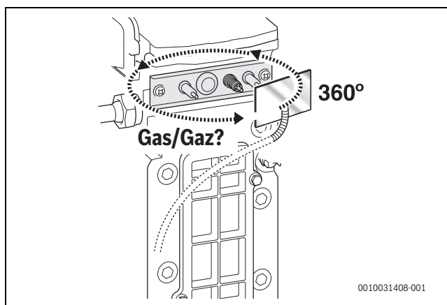
Fig. 60 Verificarea etanșeității
