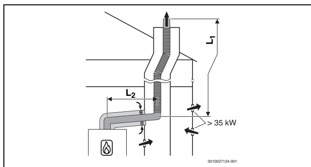
Fig. 21 Ghidarea flexibilă a gazelor arse în puț conform B 33 cu alimentare cu aer dependentă de aerul din încălț prin ghidarea concentrică a aerului/gazelor arse în încăperea centralei termice
