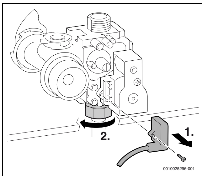
Fig. 76 Scoaterea stecker-ului și desfacerea piuliței oarbe
