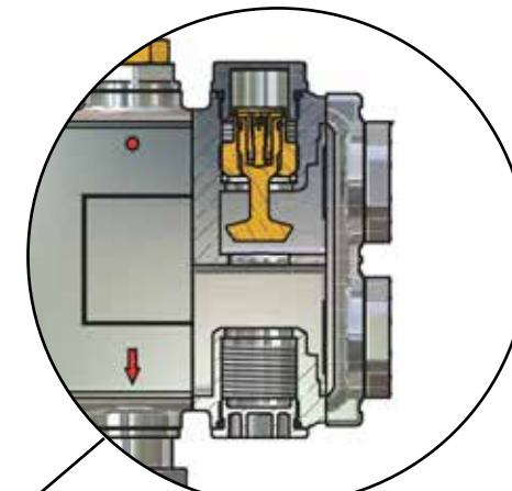
Separare hidraulică / Hydraulic separation
