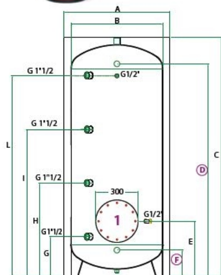
1 FLANGIA DA 200 A 2000 1 FLANGE FROM 200 TO 2000
