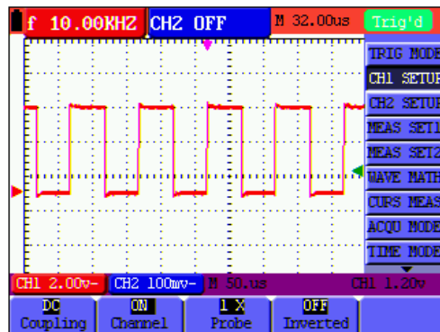
Abbildung 36: DC Kopplung
