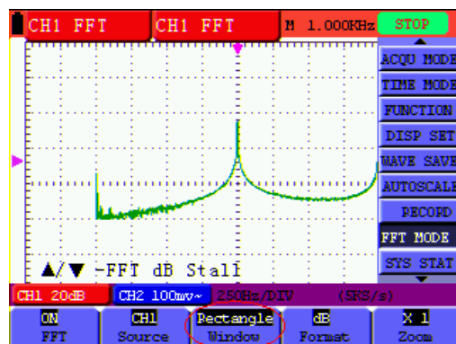
Abbildung 56: Rectangle window
