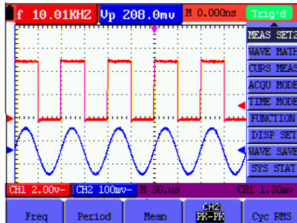
Abbildung 11: automatische Oszilloskop-Messungen
