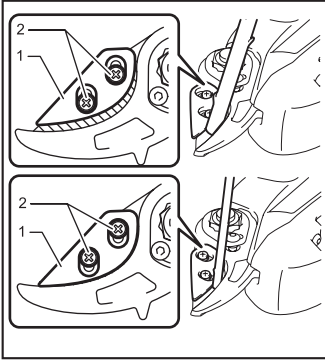
Şekil 22: 1. Tutucu 2. Vida
