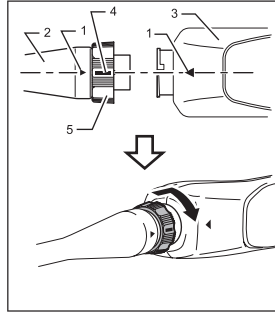
Şekil 20: 1. Üçgen işaret 2. Bağlantı kablosu 3. Makaslar 4. Kaplin üzerindeki işaret 5. Kaplin
