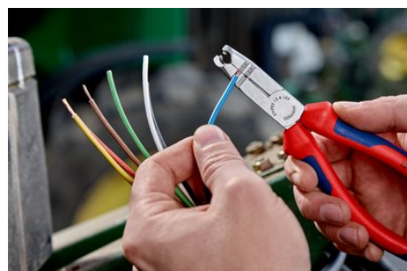
G#uri de dezizolare pentru conductori de 1,5 #i 2,5 mm 2
