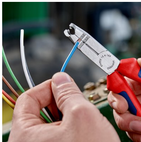
Găuri de dezizolare pentru conductori de 1,5 #i 2,5 mm²
