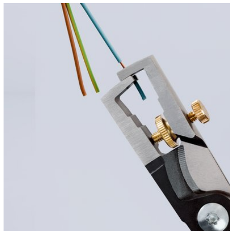
Marcaj al lungimii: marcajele optice oferã asisten#ã la dezizolãrile repetate pe lungimi comune (11 mm #i 16 mm)
