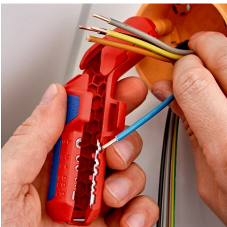
dezizolarea conductorilor individuali
