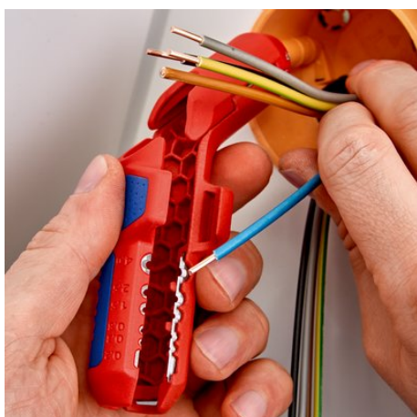
dezizolarea conductorilor individuali
