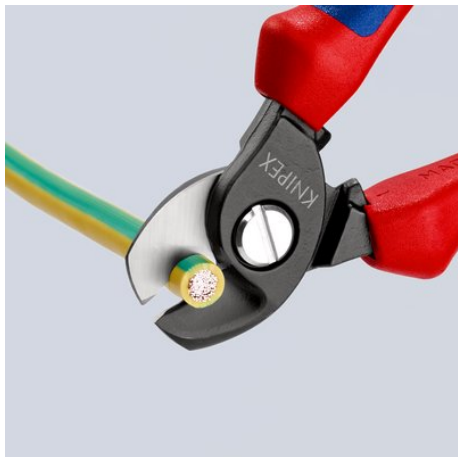
tăierea cablului lui foarfecele pentru cabluri: tăietură u#oară, fără reziduuri, fără deformarea cablului
