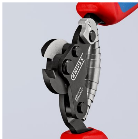
Articula#ie montată pe lagăr dublu
