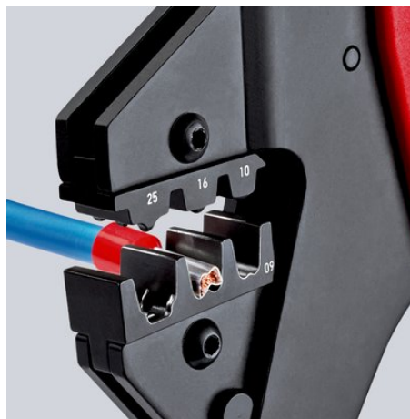
97 43 200 cu adaos de sertizare 97 49 09 pentru ferule
