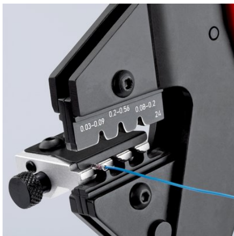
97 43 200 cu adaosul de sertizare 97 49 24 #i elementul de pozi#ionare auxiliar 97 49 93 pentru fi#e D-Sub
