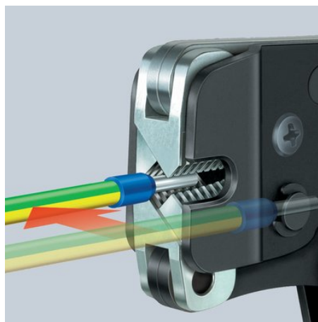
97 53 08: introducerea paralelă a ferulelor din lateral până la o adâncime de 2,5 mm 2 , de ex. în condi#ii de spa#iu strâmt
