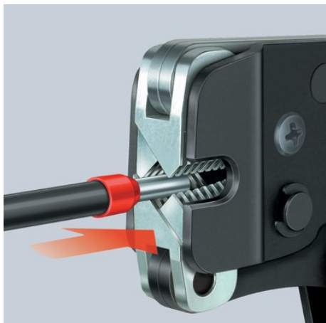
introducerea frontală a ferulelor, de ex. în tablouri electrice
