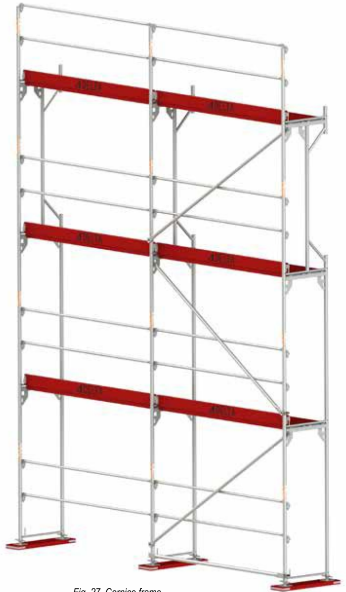
Fig. 27. Cornice frame.
