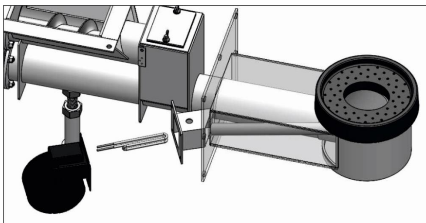
Fig 16. Înlocuirea rezistenței
