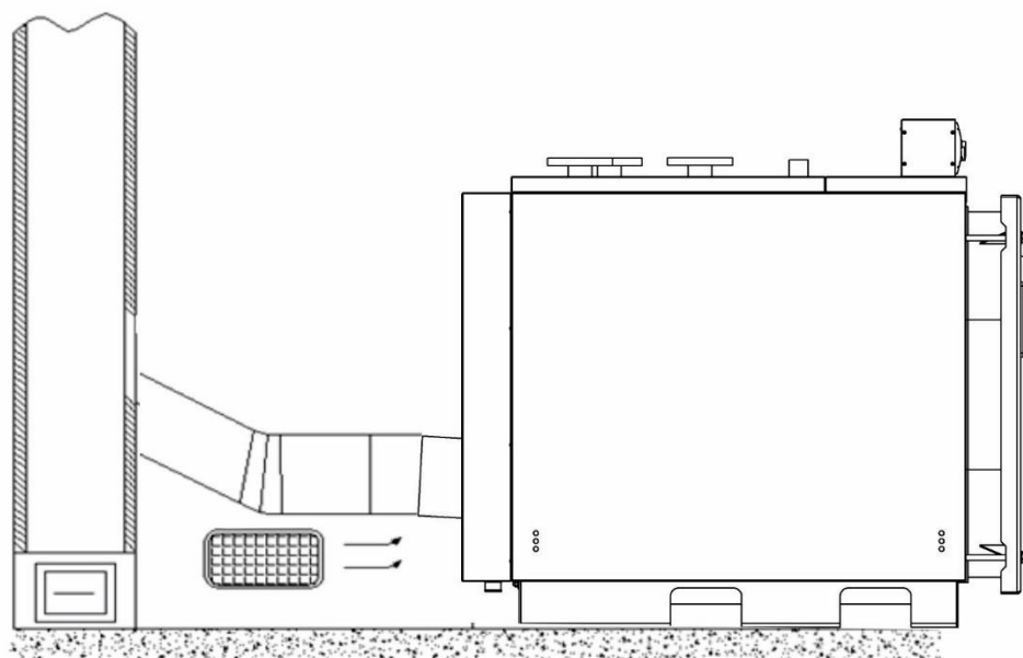
Fig 1. Camera cazanului și alimentarea cu aer
