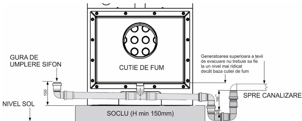
Fig 3. Drenarea condensului
