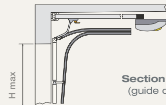
Section type A (guide unique)
