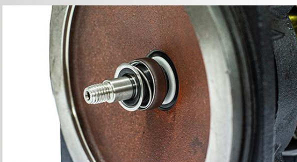
Garnitura mecanică: ceramică/grafit/NBR
