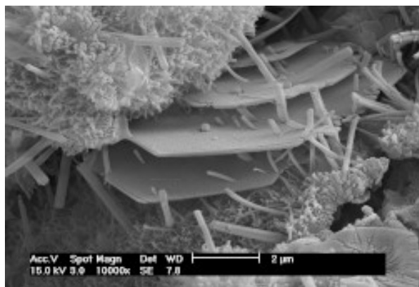
Hidratarea liantului pe baza de ciment Portland la un mortar traditional pentru rosturi
