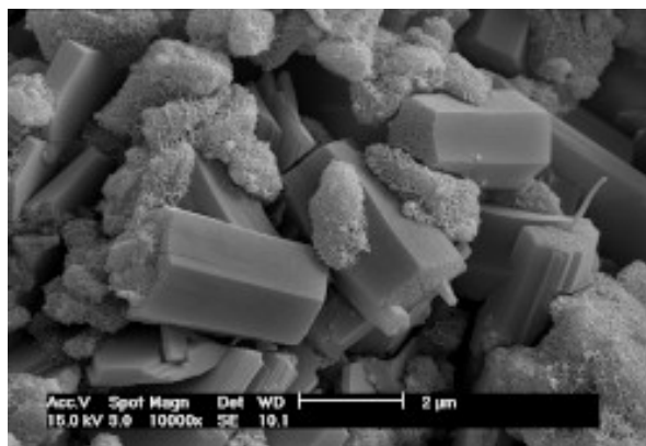
Hidratarea liantului special pe baza de ciment Ultracolor Plus. Se observa absenta cristalelor lamelare de Portlandit (hidroxid de calciu) care determina aparitia eflorescentelor
