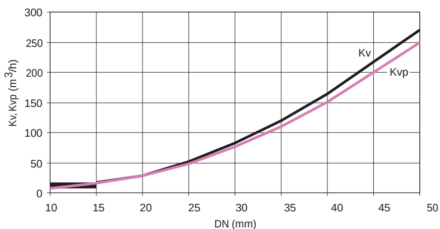
Diagrama debit-dimensiune
