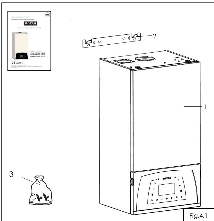
Fig. 4.1 Setul de montaj
