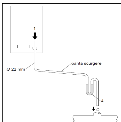
Fig. 5.5 - Eliminare condens in reseaua de canalizare
